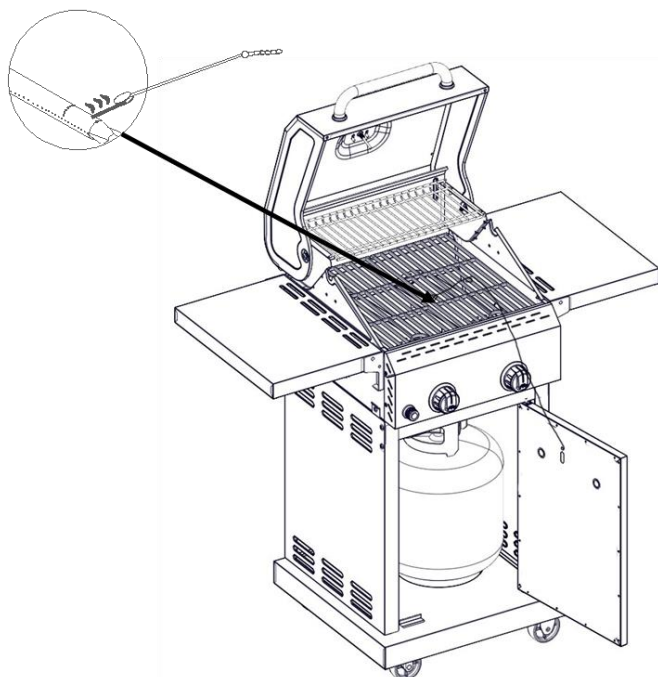
Brûleur principal
